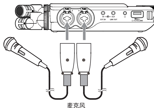
连接到输入插孔 3-4 的示例
